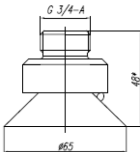
Рис. 5. Распылитель РКН-95-14,5-3/4
