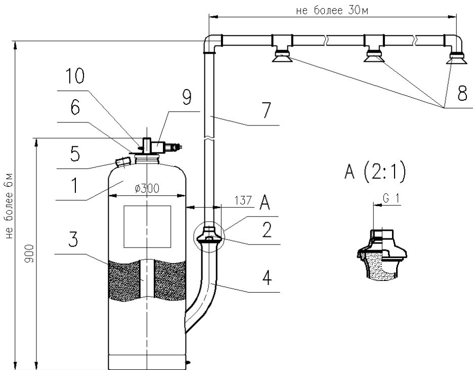
1 - корпус с огнетушащим порошком; 2 - мембранный узел; 3 - генератор газа; 4 - направляющая горловина; 5 - засыпная горловина; 6 - шильдик; 7 - трубопровод подачи порошка; 8 - распылители; 9 - узел электрозапуска; 10 - узел заземления Рис. 1 Схема модуля порошкового пожаротушения "Буран 50КД-В"
