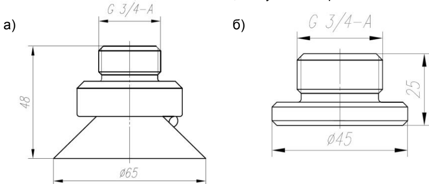
(а - РКН-95-14,5-3/4, б - РКН-19-14,5-3/4)
