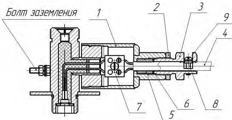
1 - муфта; 2 - гайка; 3 - штуцер; 4 - подсоединяемый кабель; 5 - кольцо уплотнительное; 6 - кольцо зажимное; 7 - клеммная колодка; 8 - планка; 9 - винт. Рис.2 Чертеж узла электрозапуска
